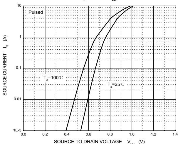
I_S — V_{SD}
