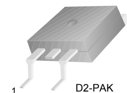
D2-PAK 1. Anode 2. Cathode 3. Anode
